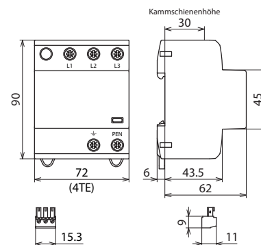
Maßbild DSH B TNC 255 FM
