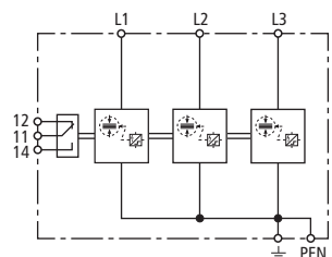
Prinzipschaltbild DSH B TNC 255 FM
