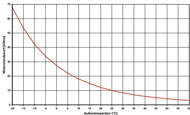
Abb. 3.3:Fühlerkennlinie NTC-10 zum Anschluss an den Heizungsregler
