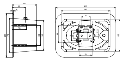
Maßbild UFTSK 7.10 FL40 300X220X120 GG
