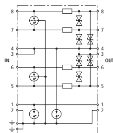
Prinzipschaltbild BVT RS485 5
