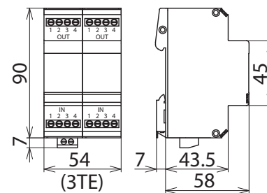
Maßbild BVT RS485 5
