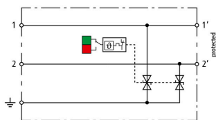
Prinzipialschaltbild BCO CL2 E 48
