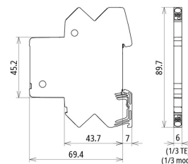
Maßbild BCO CL2 E 48
