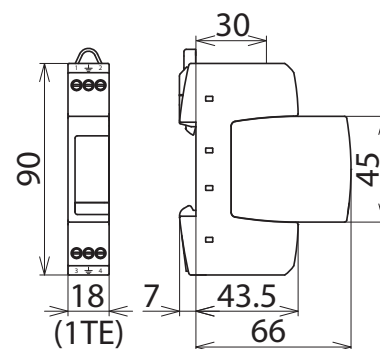
Maßbild DR M 2P 60
