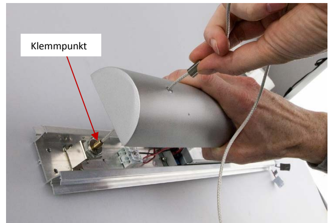
Abb. 4 - Verbindung Sekundärseite
