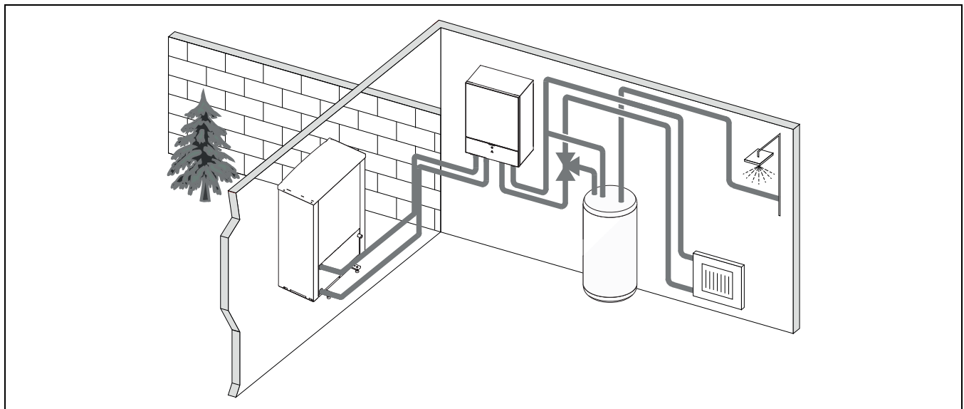
Bild 3 Wärmepumpe Compress 7001i AW, Inneneinheit AWE mit elektrischem Zuheizung und externem Warmwasserspeicher
