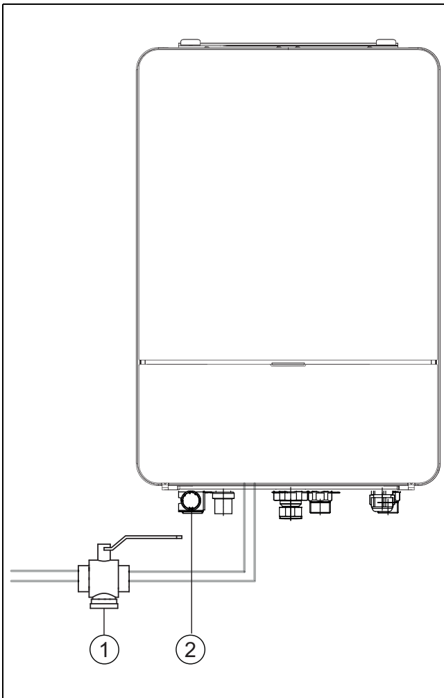
Bild 7 Inneneinheit AWE
