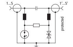
Prinzipschaltbild DGA FF5 TV
