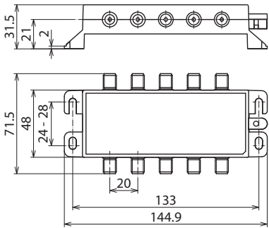
Maßbild DGA FF5 TV
