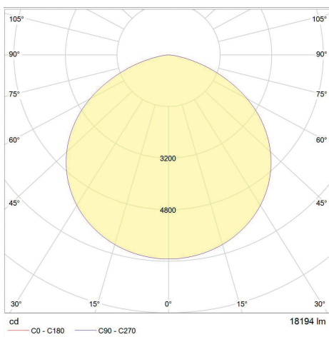
SUN 860 Polardiagramm
