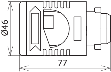
Maßbild HVI HEAD 20
