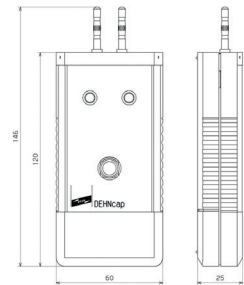
Maßbild SAG DCA A LRM
