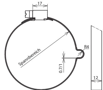
Maßbild LH 8 SB80.100 SCG V2A
