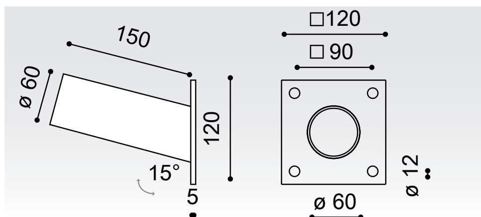
15° Wandhalterung
