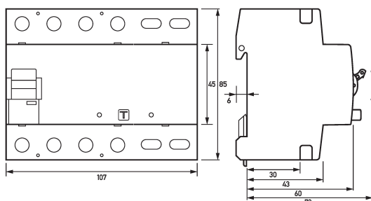
Maßzeichnung Lasttrennschalter DHS 6-063 NU
