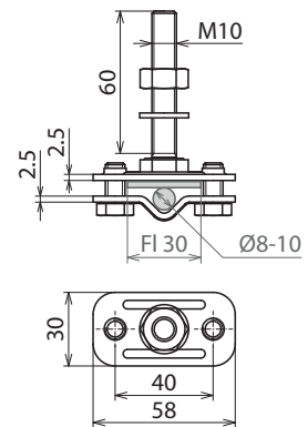
Maßbild AK ZS 8.10 FL30 GBM10X60 V4A
