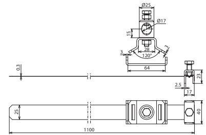
Maßbild
