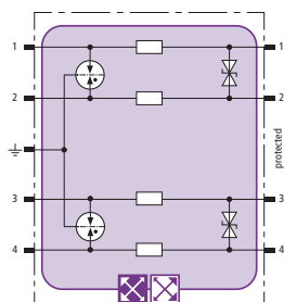
Prinzipschaltbild BXT ML4 BD 24
