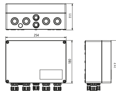
Maßbild DCU 2 YPV 1100 2M 2S
