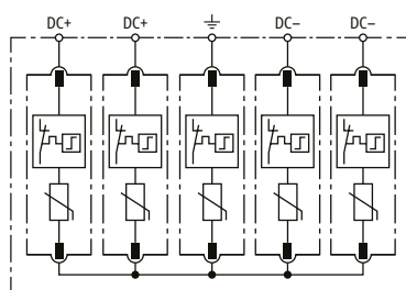
Prinzipschaltbild DCU 2 YPV 1100 2M 2S
