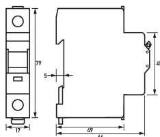
Maßzeichnung Gruppenansicht
