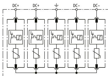
Prinzip Schaltbild DCU 2 YPV 1+2 1000 2M
