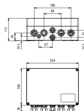
Maßbild DCU 2 YPV 1+2 1000 2M 2S FM
