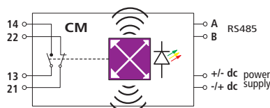
Prinzipschaltbild DRC MCM XT
