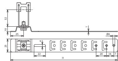
Maßbild DLH UG 8 H32 L205 V2A
