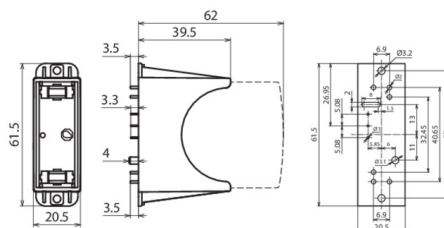
Maßbild DG PCB I 275 FM
