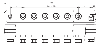
Maßbild PAS I 6AP M10 CU
