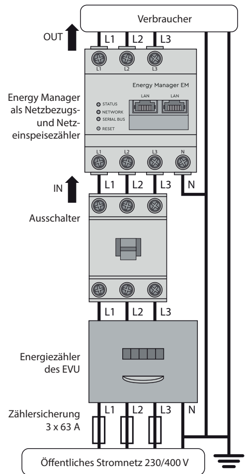
Abbildung: Anschluss bei direkter Messung
