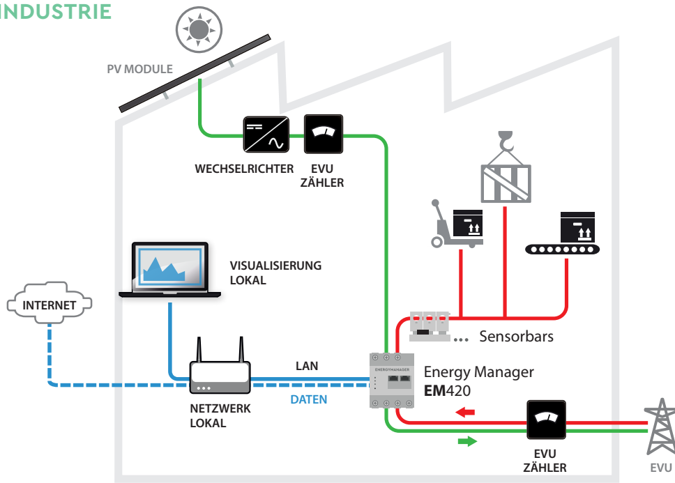
Abbildung: Anschluss bei direkter Messung
