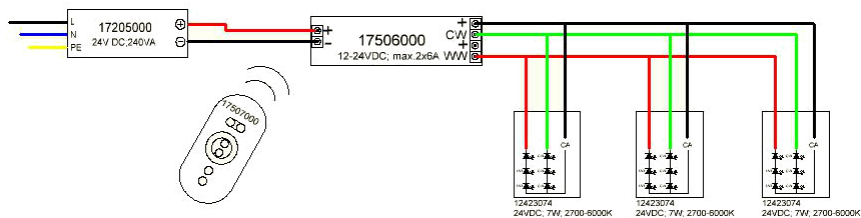
Anschlussbeispiel
