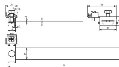
Maßbild BRS 27.60 AQ4 25 V2A
