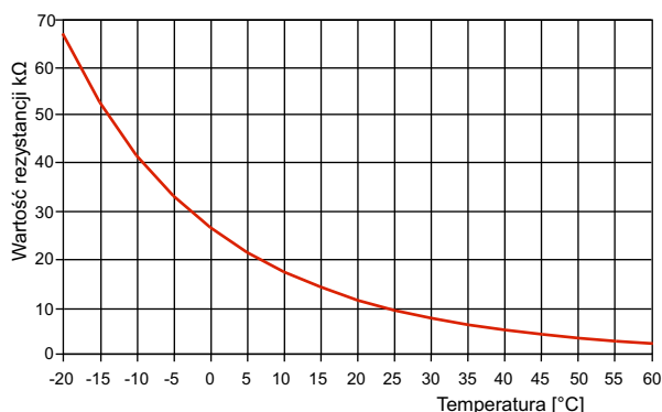
Abb. 3.3: Charakterystyka czujnika NTC-10 podłączanego do regulatora ogrzewania
