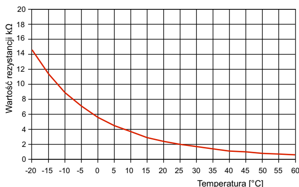
Abb. 3.4: Charakterystyka czujnika NTC-2 zgodnego z normą DIN 44574
