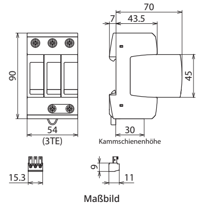
Maßbild
