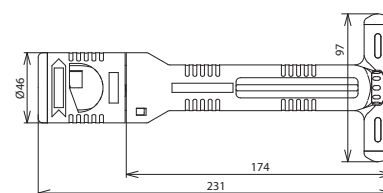
Maßbild HVI STRIP 20
