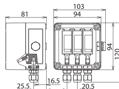
Maßbild DCU YPV SCI 1000 1M
