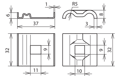
Maßbild KP AQ4 50 DUL 8.10 VKL9 V2A
