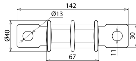
Maßbild DSFS
