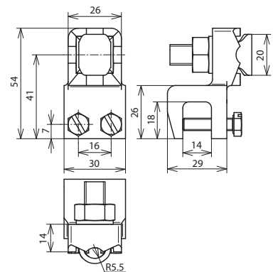
Maßbild AK 7.10 KSV KBF1 12 TGTZN
