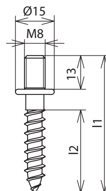
Maßbild HSC 8X42 AGM8X13 STGALZN
