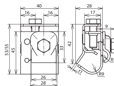
Maßbild DRK KB 6.10 W16.22 STTZN
