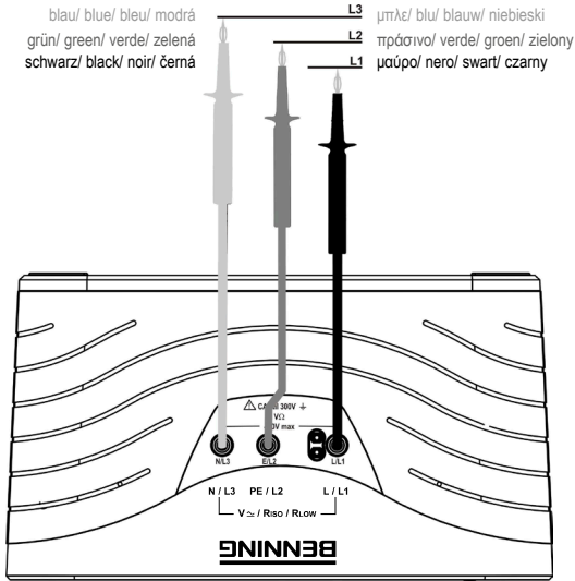
Bild 7: Drehfeldprüfung (Phasenfolge) Figure 7: Rotary field (phase sequence) Fig. 7: Test d'ordre de phases Figura 7: Verifica della sequenza di fase (sequenza fasi) Fig. 7: Roterende veldtest (fasevolgorde)
