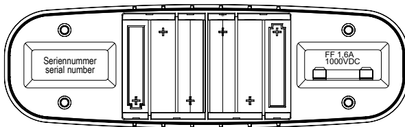
Bild 8: Batterie-/ Sicherungswechsel Figure 8: Battery/fuse replacement Fig. 8: Remplacement des piles et du fusible Figura 8: Sostituzione batterie / fusibili Fig. 8: Batterijen zekering vervangen
