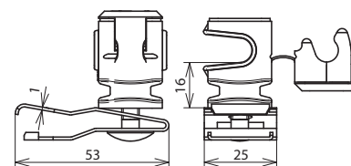
Maßbild LH FS 8 H16 GR V2A
