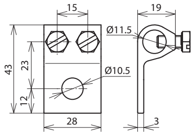
Maßbild KS 7.10 B10.5 AL
