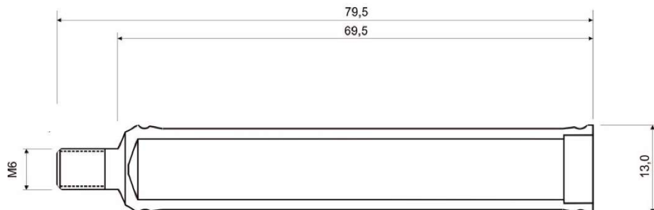
Seitenansicht (Schnitt)
