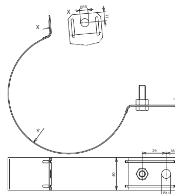
Maßbild RRS 120 B11 STTZN
