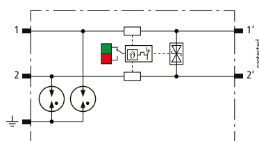
Prinzipschaltbild BCO ML2 BD HF 5
