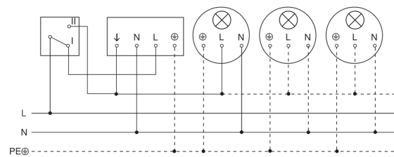
Schaltplan Anschluss 4-fach Tasterkoppler an DALI2 APC
