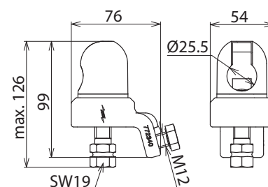
Maßbild KKH 25 D SK
