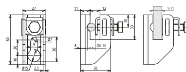
Maßbild FRH 11 6.10 WA11 B7 STTZN
