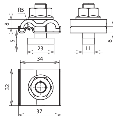
Maßbild UEK 8.10 AQ4 50 HKSM10 V2A
