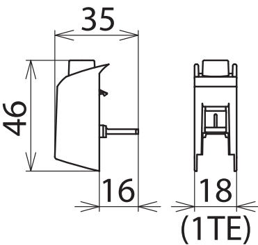
Maßbild STAK 25
