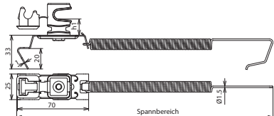
Maßbild DLH SSL 8 H16 FG180.280 GR V2A
