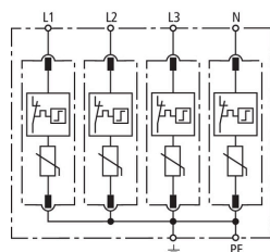
Prinzipialschaltbild DG M TNS 385
